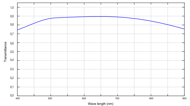
Transmission 分光透過率
